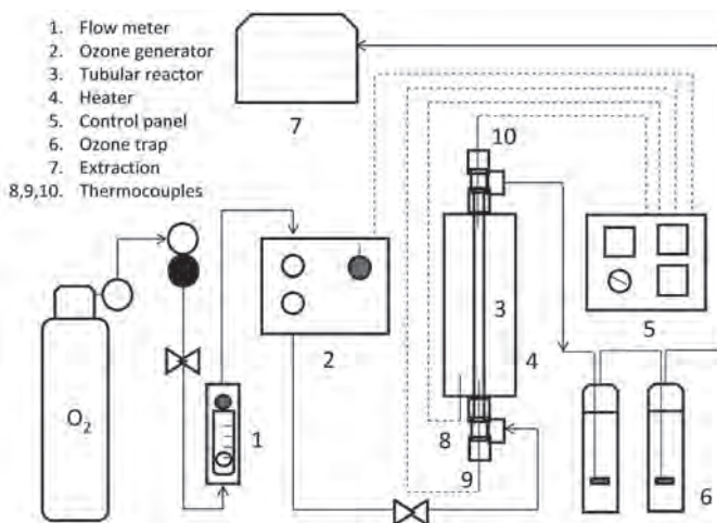
รูปที่ ๑ แสดงรายละเอียดและการติดตั้งอุปกรณ์การทดลอง
