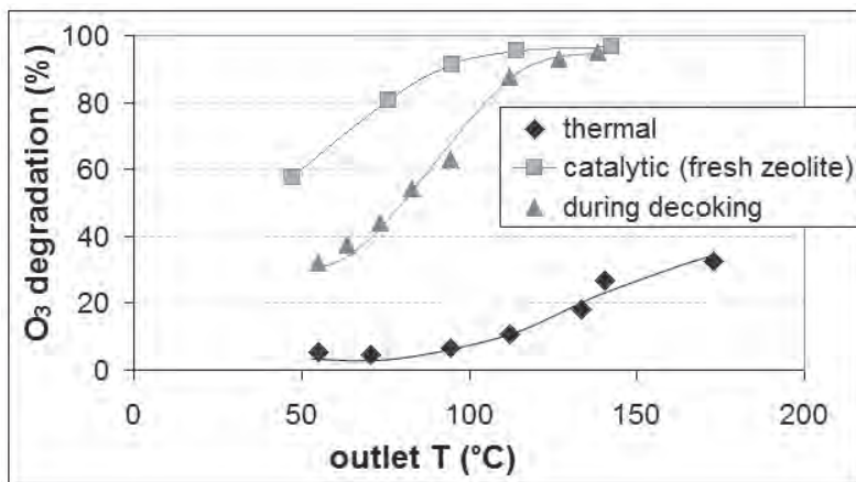
รูปที่ ๖ การสลายของโอโซนที่อุณหภูมิต่าง ๆ ปริมาณการไหล ๑๒.๗ ลิตรต่อชั่วโมง ความเข้มข้น ๔๘ กรัมต่อลูกบาศก์เมตร
