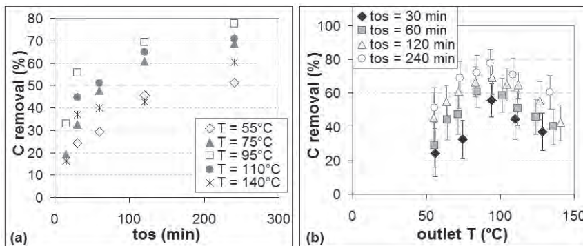
รูปที่ ๗ ประสิทธิภาพการฟื้นฟูตัวเร่งสัมพัทธ์กับ (a) เวลาการดำเนินงาน (b) อุณหภูมิของแก๊สขาออก ที่อัตราการไหลของแก๊ส ๑๒.๗ ลิตรต่อชั่วโมง ความเข้มข้นของโอโซน ๔๘ กรัมต่อลูกบาศก์เมตร
