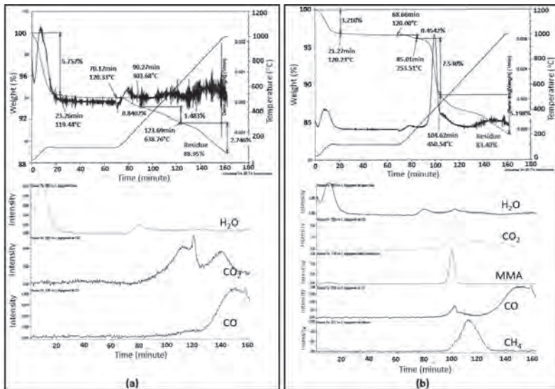
รูปที่ ๔ Thermograms ของแก๊สที่เกิดขึ้นในเครื่อง IR Spectroscopy
