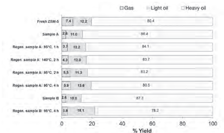
รูปที่ ๑๑ ผลิตภัณฑ์ที่ได้จากการสลาย PMMA ด้วยตัวเร่งที่ผ่านการฟื้นฟู
