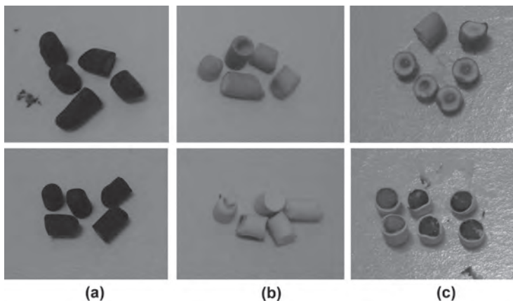
รูปที่ ๙ ภาพตัวเร่งปฏิกิริยา (a) มีถ่านโค้กติดอยู่ (b) ผ่านการฟื้นฟู (c) ถูกผัดรีงทำการทดลอง ที่ปริมาณการไหลของแก๊ส ๑๒.๗ ลิตรต่อชั่วโมง เวลา ๑ ชั่วโมง แฉวบน อุณหภูมิ ๑๐๐ องศาเซลเซียส แฉวล่าง อุณหภูมิ ๑๔๐ องศาเซลเซียส
